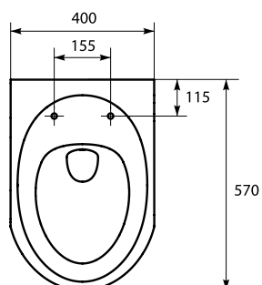
OK-03-002 Miska zawieszana BILBAO Rozmiar: szerokość 40; wysokość 37; głębokość 57/ BILBAO wall hung bowl width 40; height 37; depth 57
