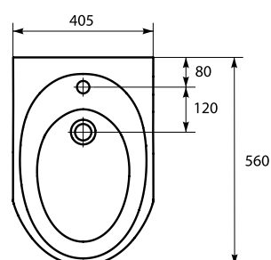
OK-03-001 Bidet zawieszany BILBAO Rozmiar: szerokość 40,5; wysokość 34,5; głębokość 56/ BILBAO wall hung bidet width 40,5; height 34,5; depth 56
