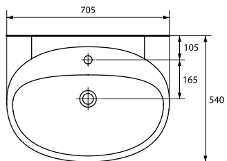
OK-02-001 Umywalka KIOTO 70 z otworem na armaturę, montaż na szafce lub z półpostumentem Rozmiar: szerokość 70,5; wysokość 21; głębokość 54/ KIOTO 70 washbasin with hole for mixer, assembly with a semi-pedestal or on a countertop. width 70,5; height 21; depth 54
