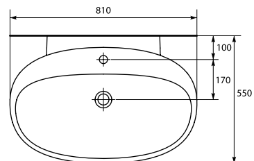
OK-02-002 Umywalka KIOTO 80 z otworem na armaturę, montaż na szafce lub z półpostumentem/ Rozmiar: szerokość 81; wysokość 20,5; głębokość 55/ KIOTO 80 washbasin with hole for mixer, assembly with a semi-pedestal or on a countertop. width 81; height 20,5; depth 55
