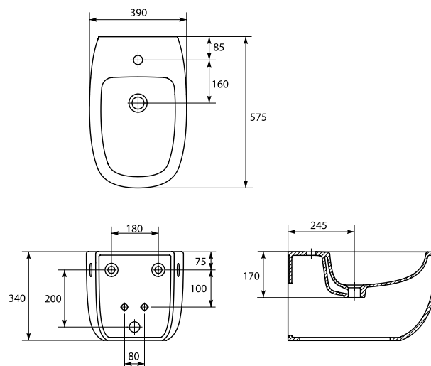
OK-02-005 Bidet zawieszany KIOTO Rozmiar: szerokość 39; wysokość 34; głębokość 57,5/ KIOTO wall hung bidet width 39; height 34; depth 57,5
