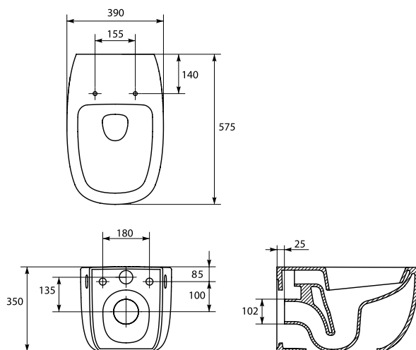
OK-02-006 Miska zawieszana KIOTO Rozmiar: szerokość 39; wysokość 35; głębokość 57,5/ KIOTO wall hung bowl width 39; height 35; depth 57,5
