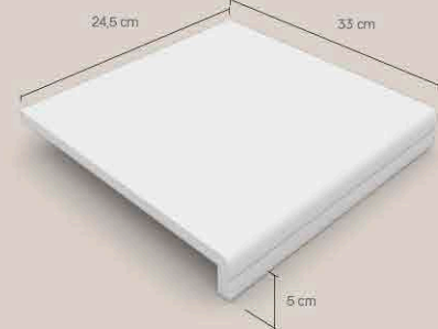
PELDAÑO RECTO T-4 T-4
